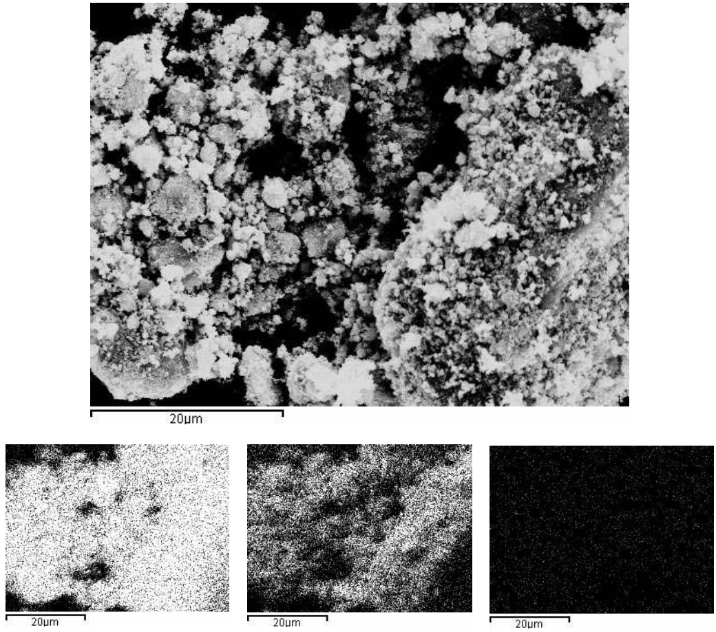
Fig. 35: TiLi(5)W(5) (a) and Titanium (b), Oxygen (c), Tungsten (d) mapping.
